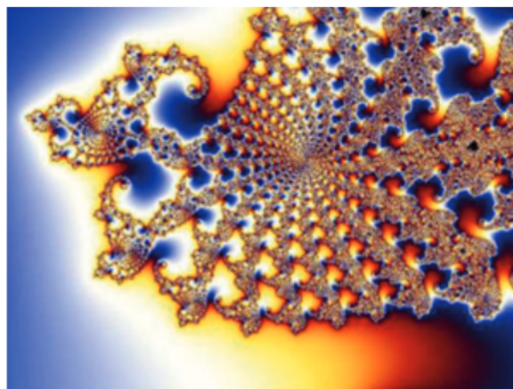
Ejemplo de fractal.
